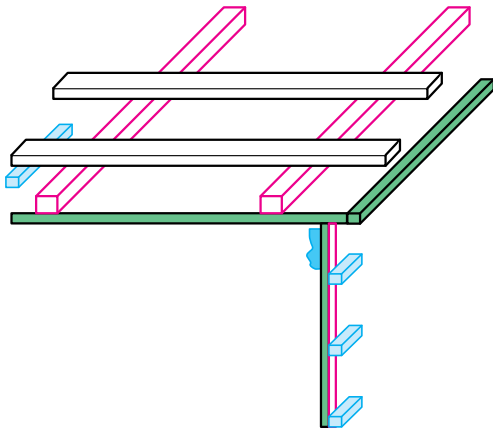
شکل ۷-۴۱- استفاده از L یا گونیاى ۹۰ درجه برای چسباندن چوب‌های شیب‌دار
