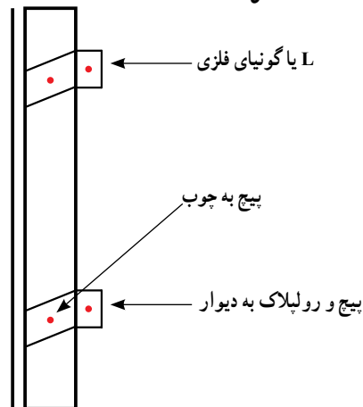
شکل ۳۰-۷ استفاده از L یا گونبای ۹۰ درجه برای چسباندن چوب‌های شیب‌دار
