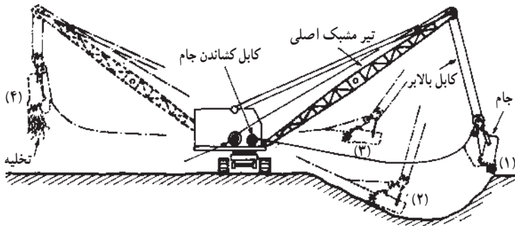
شکل ۲۶-۴- نحوه گودبرداری به وسیله دراگ‌لین
