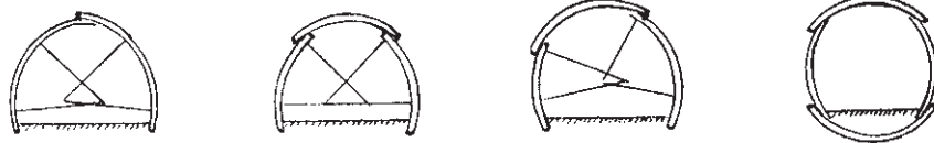
شکل ۶-۲۵- انواع قاب های کشویی چند تکه ای
