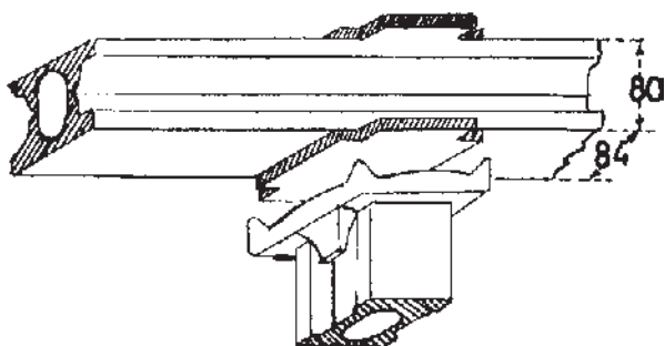
شکل ۱۲-۲۷- دستک لوله متشکل از ۲ نیم ناودانی
