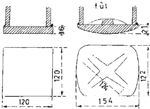
شکل ۱۱-۲۶- سینی
