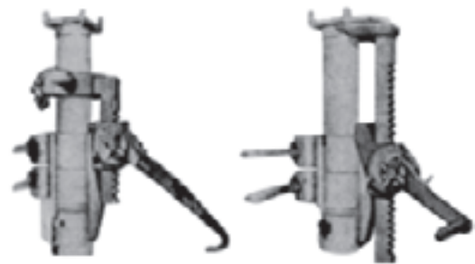
شکل ۸-۲۶- کشنده‌ی کشویی
