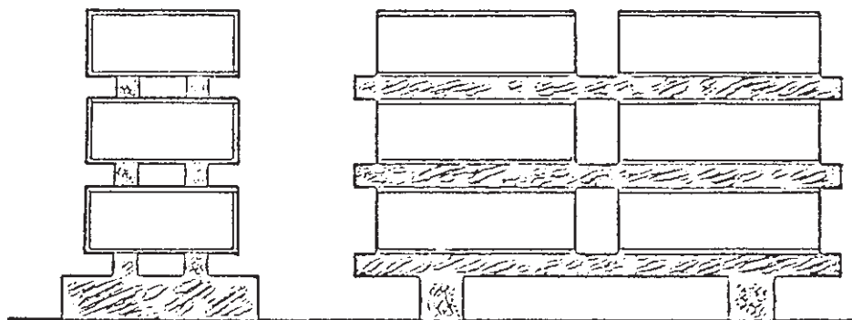
شکل ۳-۹- طرز چیدن کارتن‌های مواد منفجره در انبار
