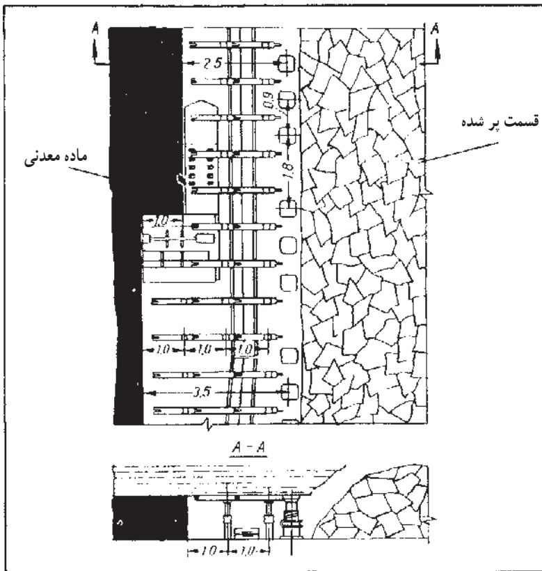
شکل ۹-۲- وضعیت کلی کارگاه استخراج [۳۲]
