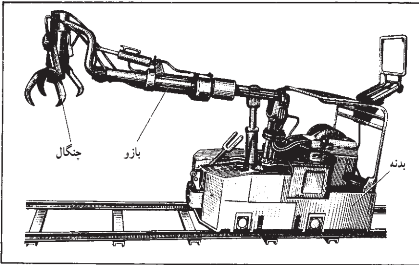
شکل ۷-۳۰- ماسین نصب بلوک‌های سنگین [۲۳]
