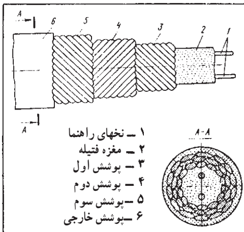
شکل ۱۱-۵- فتیله انفجاری (۸)
