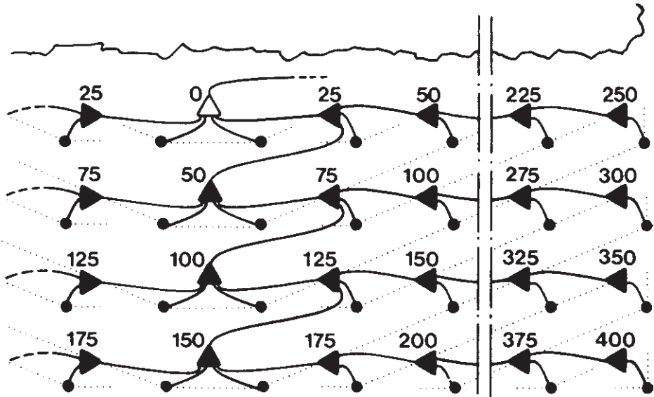
شکل ۲۱-۵- ارتباط مدار آتشکاری پله با نانل یونیدت
