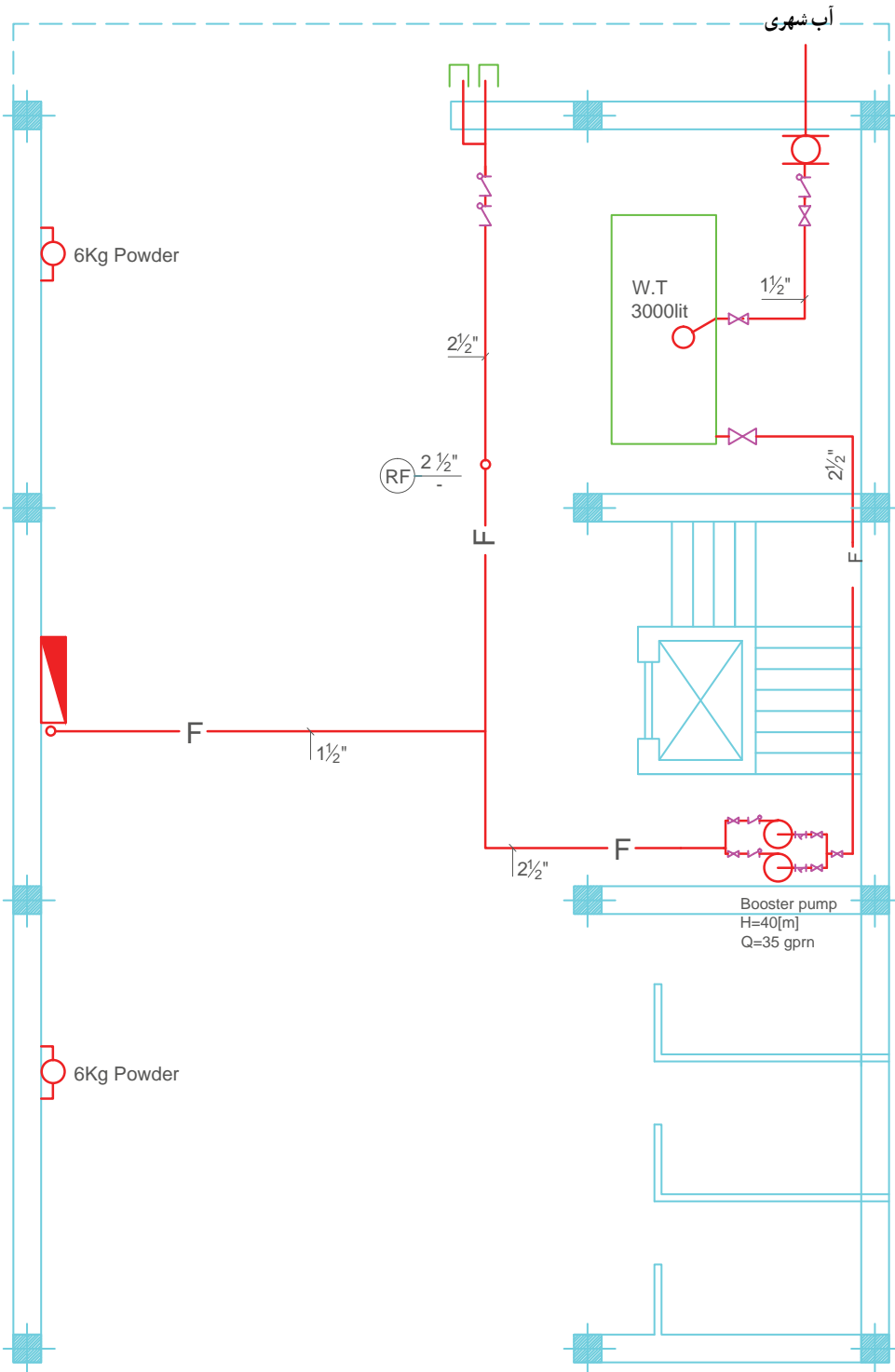
شکل ۳-۴ - الف - پلان لوله کشی آب آتش نشانی طبقه همکف - مقیاس ۱/۱۰۰
