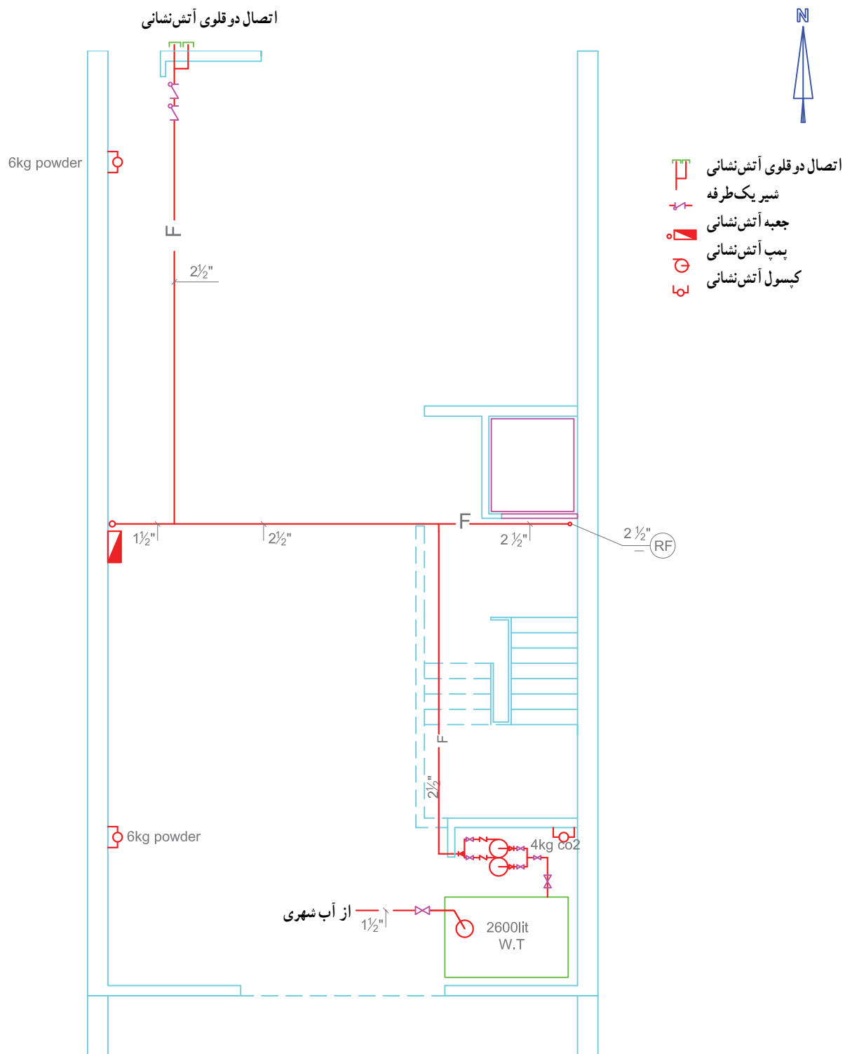
شکل ۲-۴- الف- پلان لوله‌کنشی آب آتش نشانی طبقه همکف- مقیاس ۱/۱۰۰
