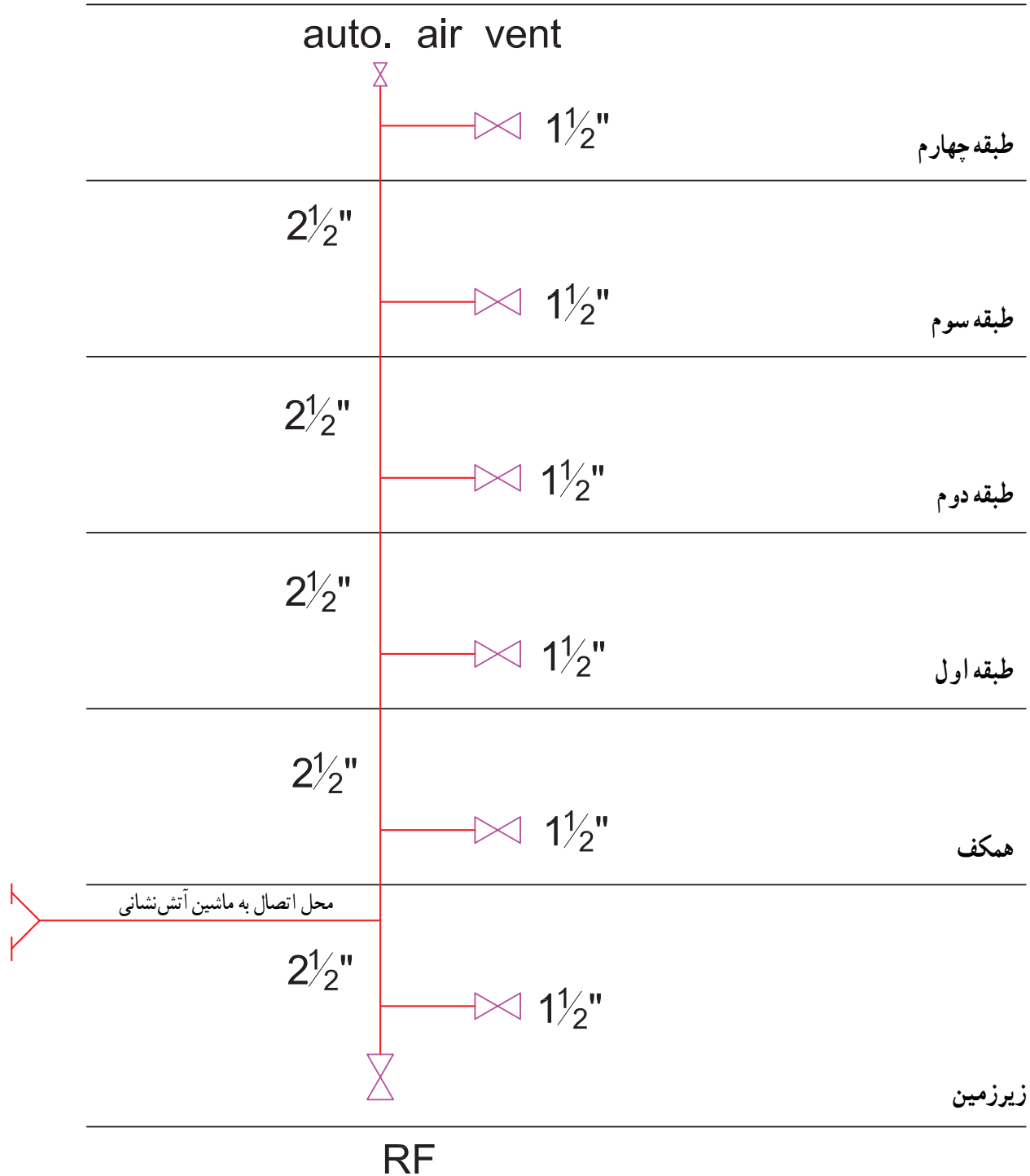
شکل ۱-۴-۱- ت- رایزر دیگرام لوله‌کشی آتش‌نشانی - مقیاس \frac{1}{100}
