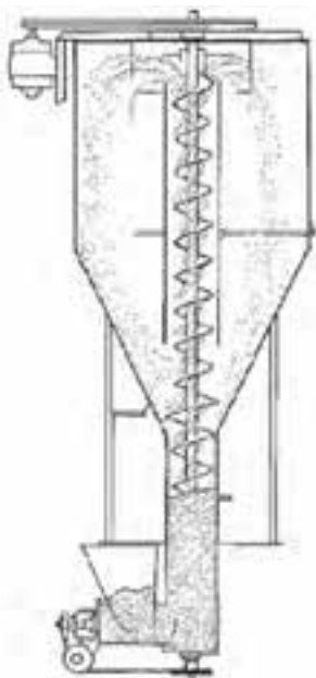
شکل ۴-۳ میکسر عمودی
