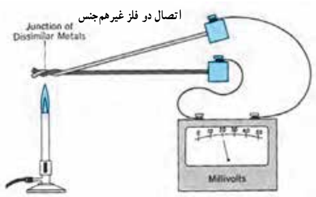
ترموکوپل گرم شده توسط شعله‌ی ۲۰ mv برق تولید می‌کند.
