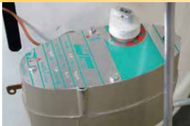
شکل ۱-۵۲- قرار دادن کلید گردان در حالت خاموش
