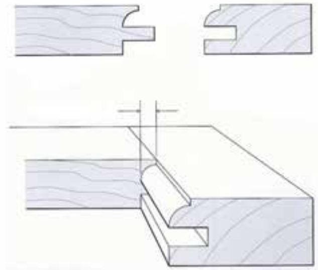
شکل (۵-۳۸) اتصال فاق و زبانه با فرز و تیغه مخصوص برای قاب پروفیل شده در نما و تصویر مجسم
