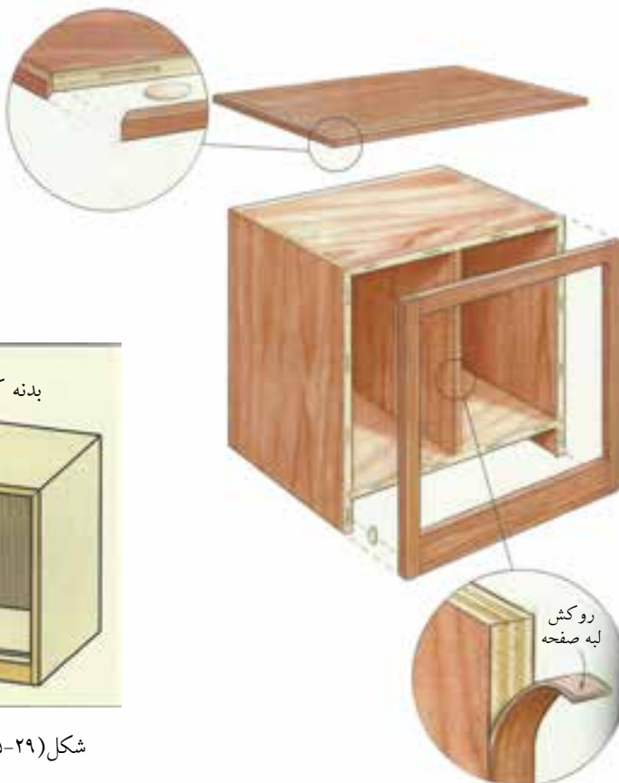
شکل (۵-۲۸) تصویر مجسم کابینت با اتصال نما با قاب و اتصال بیسکویتی
