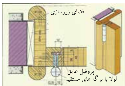
قید قاب دوراھه شده
