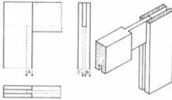
شکل ۶۱-۵: ترسیم اتصال گوشه‌ای فاق و زبانه با برکج در سه نما و تصویر مجسم به مقیاس ۱:۵
