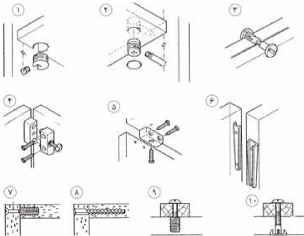
شکل (۵-۵) موارد ۱ تا ۱۰ انواع اتصالات جداشونده به وسیله یراق‌ها و پیچ و مهره برای اتصال صفحات کابینت‌ها و قطعات تختخواب و مصنوعات چوبی
