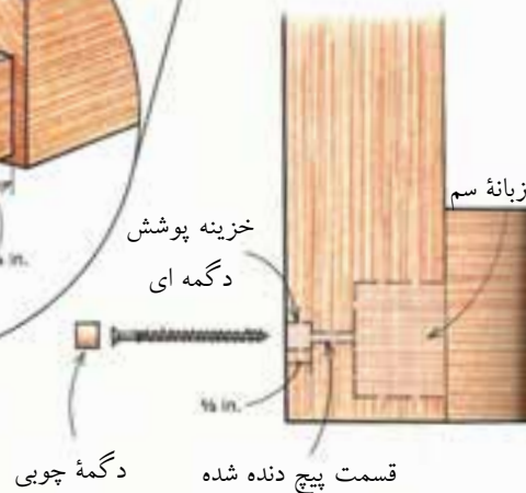
شکل (۵-۳۲) اتصال گوشه‌ای کم و زبانه با پیچ و پوشش دگمه‌ای برای درها با نمای کرکره‌ای با تصویر انفجاری
