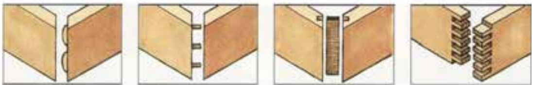
شکل (۵-۴۷) اتصال گوشه‌ای تصویر مجسم اتصالات انگشتی، قلیف زبانه جدا، دوپل و بیسکویتی
