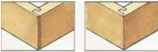
شکل (۵-۴۴) نیم و نیم دورو فارسی با دوپل اتصال قلیف زبانه سرخود
