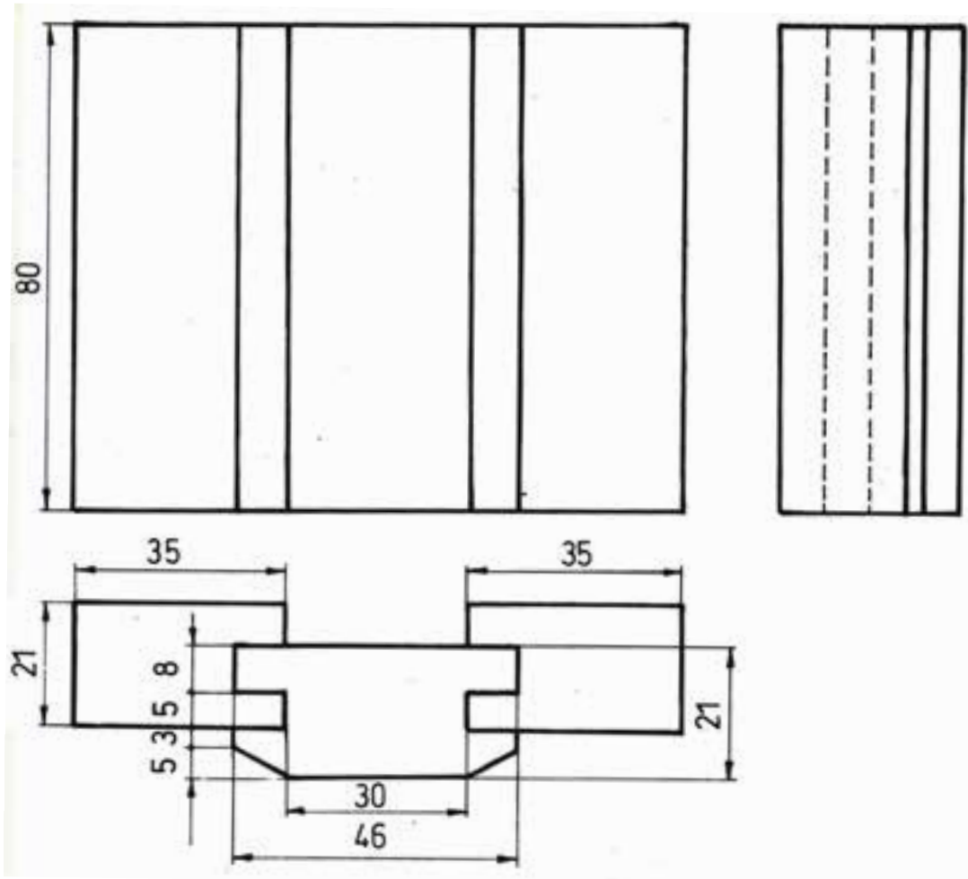
شکل (۱۰۰-۵) ترسیم اتصال عرضی به وسیله کنشکاف قیدهای به هم متصل شده در سه نما (قلیف زبانه سرخود) با اندازه گذاری
