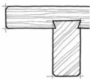
شکل (۵-۱۰۴) ترسیم اتصال گرات دو طرفه ۱:۱ M
