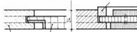
شکل (۵-۱۱۵) ترسیم اتصال قاب و تنکه هشت نوع مختلف صفحه‌چوبی تنکه از صفحات چندلایي با صفحه‌چوبی و قاب چوبی تنکه دوراهه شده با پوشش فلزی
