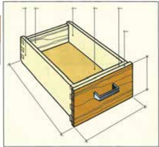
شکل (۵-۴۲) تصویر مجسم با اتصالات گوشه‌ای
