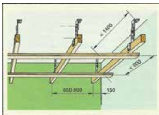
شکل (۱۲۱-۵) تصویر مجسم اتصال یراق از جنس مواد مصنوعی لولایی مخصوص زیرسازی سقف کاذب
