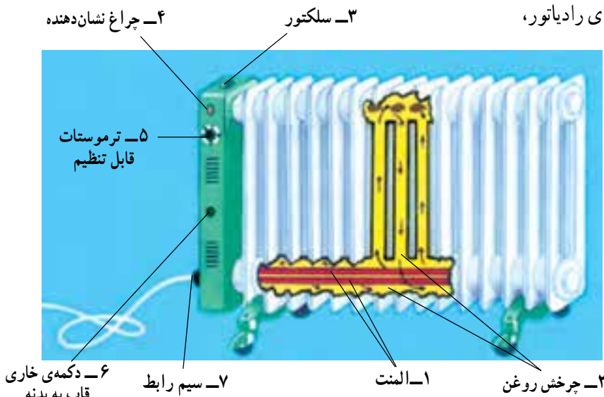
شکل ۴-۱۷ رادیاتور برقی با چرخش روغن
