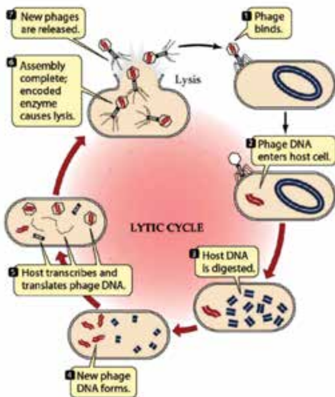
شکل ۳-۶ چرخه لیتیک زندگی باکتریوفاژ
