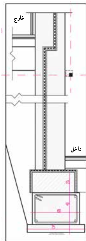
شکل ۲۰-۸ - مقاطع پلان کرسی چینی
