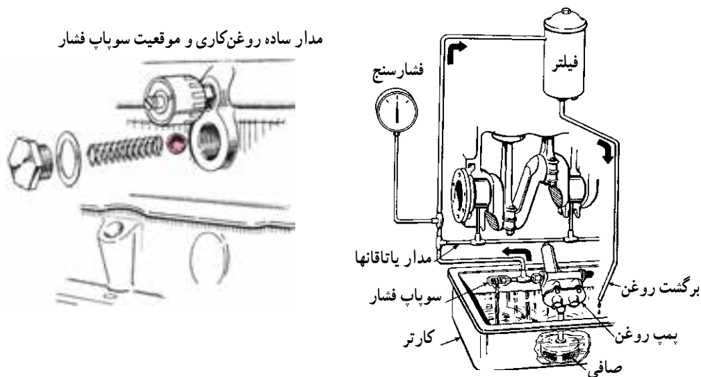
شکل ۱-۶- وقتی فشار مدار زیاد شود ساچمه فنر را فشرده کرده و مدار روغن را به کارتر باز می کند.
