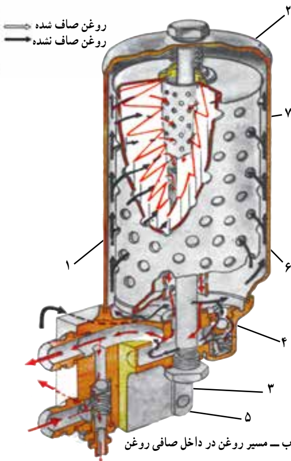
شکل ۱۲-۶ - مسیر روغن
