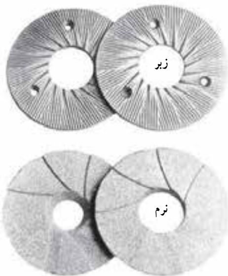
شکل ۳۸-۳- سنگ آسیا
