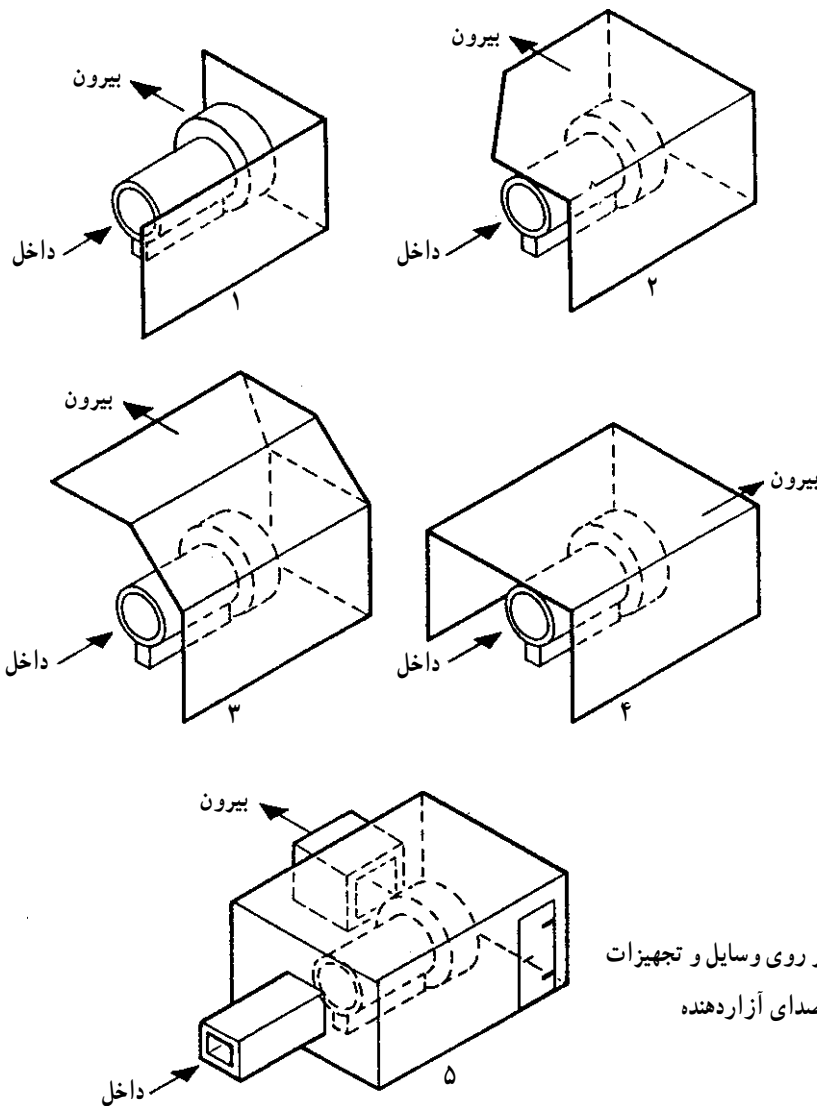
شکل ۳-۷ - کنترل صدا
