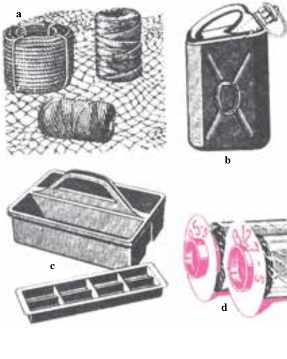
شکل ۱-۳- کاربرد انواع ترموپلاست ها
