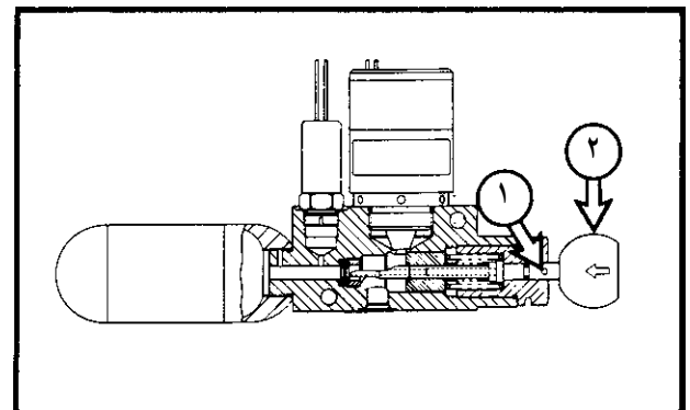
شكل ۴۰-۴- سيستم اطفای حریق
