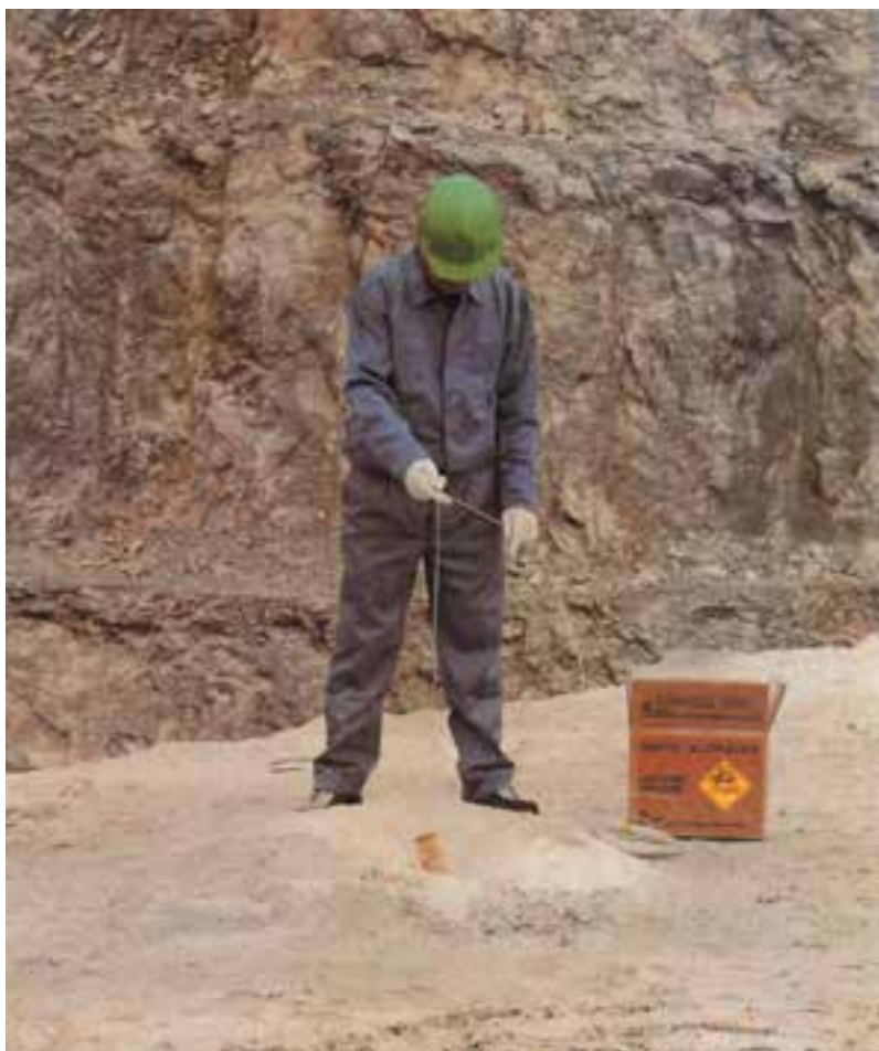
شکل ۸-۱۲- خرج گذاری پرایمر در چال با فتیله انفجاری
