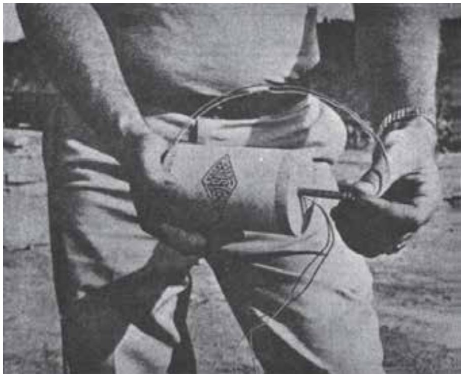
شکل ۸-۱۱ - قرار دادن چاشنی برقی در پرایمر
