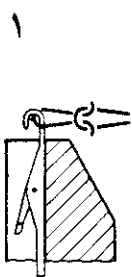
شکل ۱۱-۱۷- نمای داخلی از یک ابزار ماشین گردباف و تنظیم بادامک بالابرنده در سه موقعیت نبافت، نیم بافت و بافت
