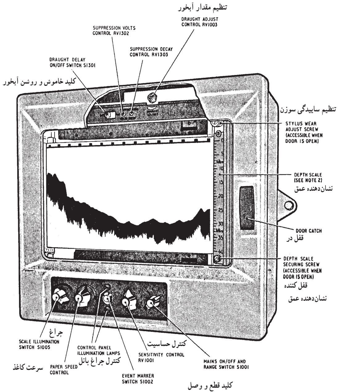
شکل ۱۰-۶- ثبت کننده عمق یاب
