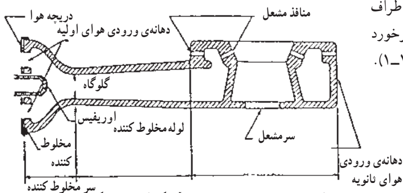
شکل ۱-۱۱۱- روشن شدن مشعل آب گرمکن مخزنی گازسوز
