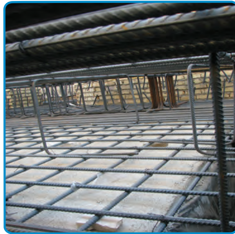
شکل ۳-۵۳- استفاده از خرک در میلگرد گذاری پی
