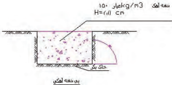
شکل ۳-۳۲ پی شفته آهکی
