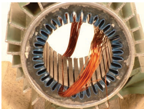
شکل ۲-۱۰- طول کاغذ پرشمان از هر طرف شیار حدود ۲ تا ۲/۵ میلی‌متر بیشتر است.
