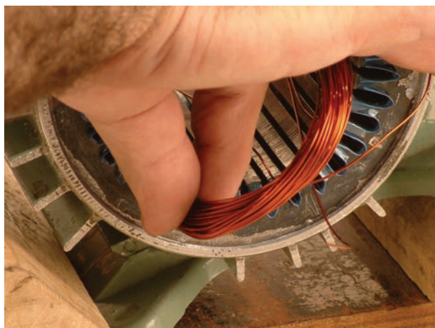
شکل ۲-۱۵- قراردادن بازوی شماره یک در شیار شماره ۱
