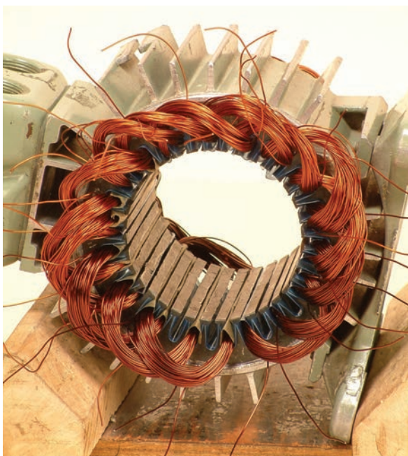
شکل ۲-۳۴- موقعیت کلاف‌ها از کلاف شماره ۱ تا کلاف شماره ۱۶
