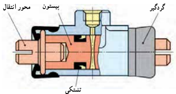
شکل ۱-۳۶- سیلندر ترمز چرخ کفشکی
