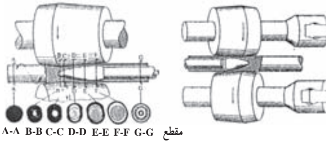
شکل ۱۰-۵- تولید لوله بدون درز توسط مغزی گذاری
