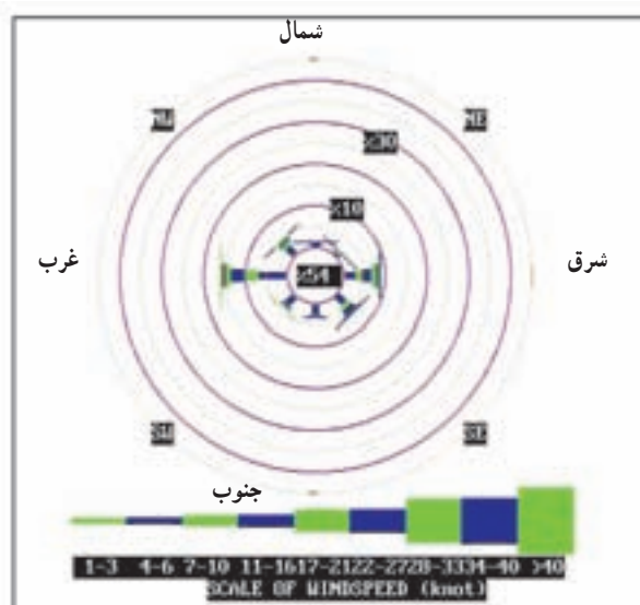
شکل ۲۷-۱. نمودار گلباد شهر ایلام
