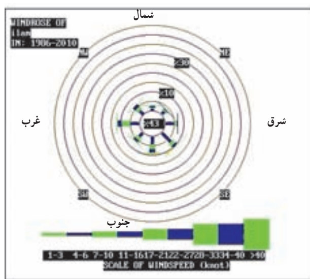
شکل ۲۸-۱. نمودار گلباد شهر دهلران
