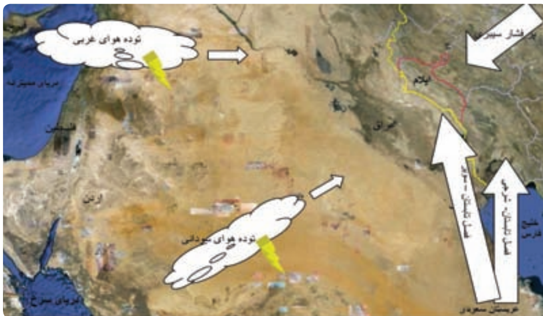
شکل ۲۰-۱- توده هوای تأثیرگذار در استان ایلام
