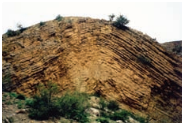
شکل ۱۰-۱- چین قائم در جاده خوش بیلاق در مسیر آزادشهر - شاهرود
