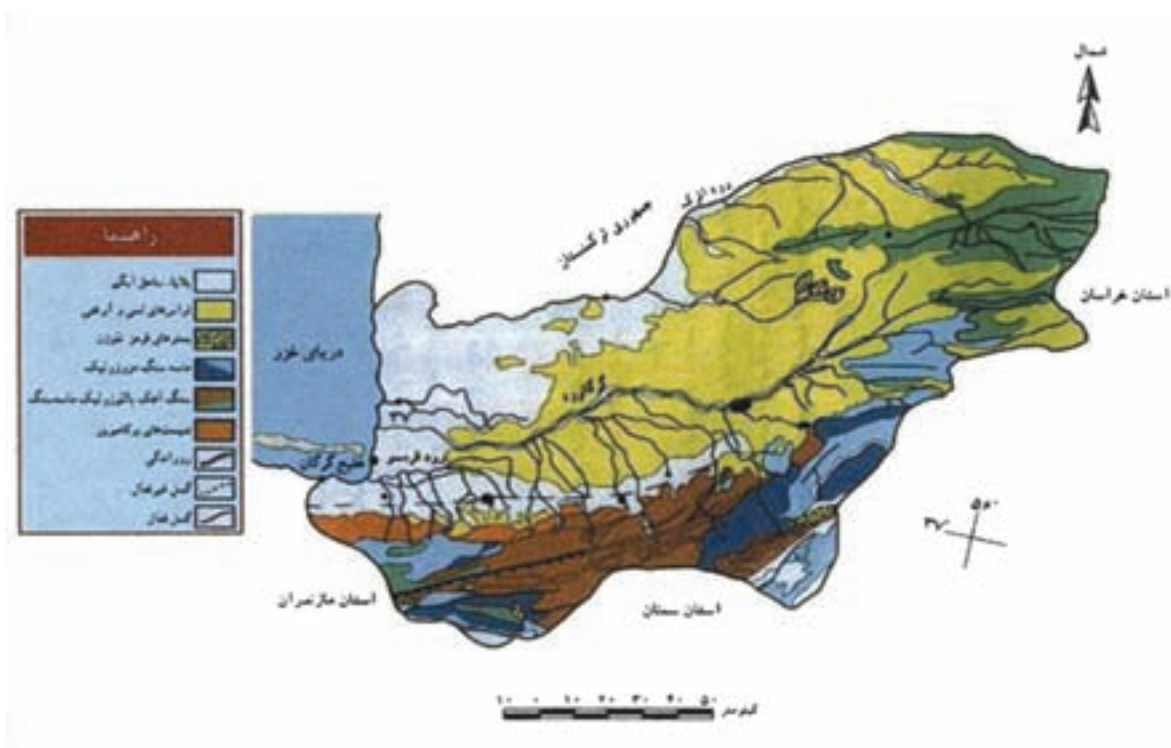
شکل ۱-۲- نقشهٔ زمین‌شناسی استان گلستان
