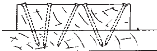
شکل ۵-۷۴- کوبیدن میخ به صورت دم چلچله
