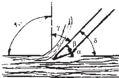
α: زاویه قرار β: زاویه گوه δ: زاویه برش
