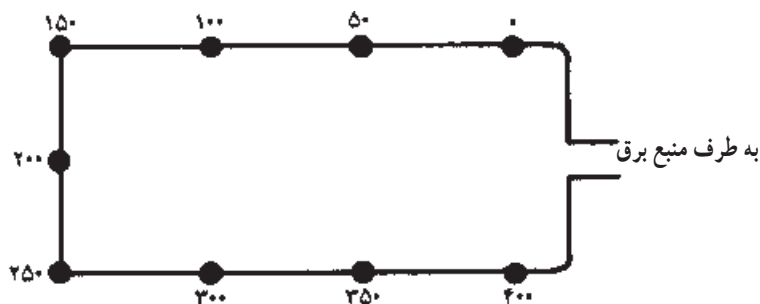
شکل ۷-۵۱- انفجار تعدادی چال با فاصله زمانی ۵۰ میلی ثانیه به وسیله چاشنی برقی کم تأخیری. چون تعداد چاشنی‌ها محدود است تعداد چال‌ها نیز محدود خواهد بود.
