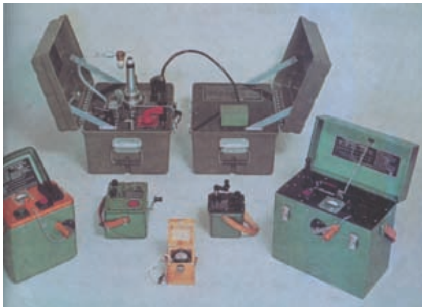
شکل ۷-۴۶- چند نوع ماشین آتش کن برقی ۱ ساخت نیترو نوبل
