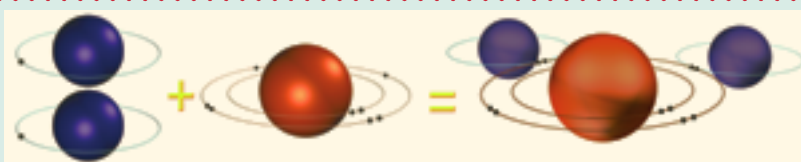
مولکول آب ( H_2O ) یک اتم اکسیژن ( O ) دو اتم هیدروژن ( H )
